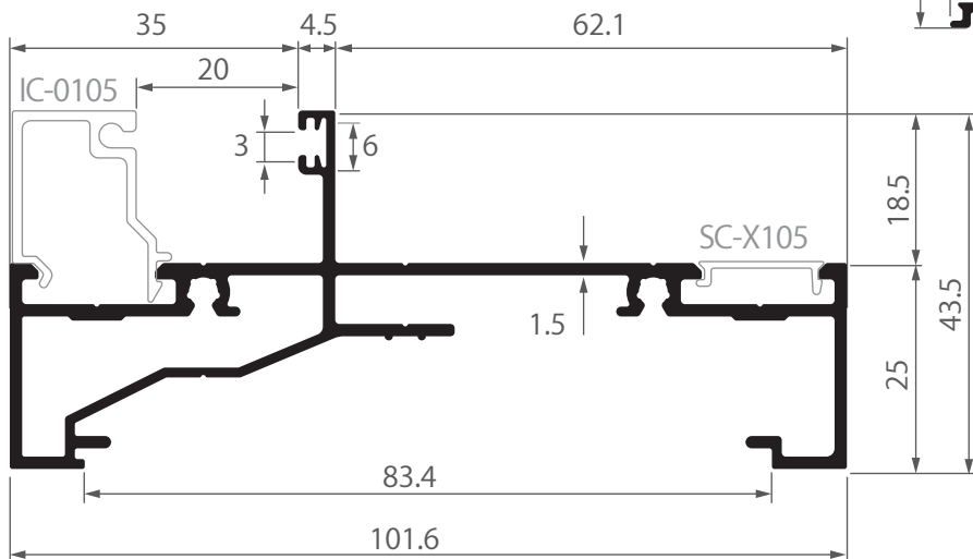
SC-X106 เสริมช่องแสงเฟรมบานกระทุ้ง สمارท เอ็กซ์ 0.426 kg/m
