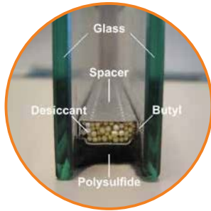
เครดิตภาพ : The constructor ภาพแสดงการส่วนประกอบ ของกระจกอินซูลา
