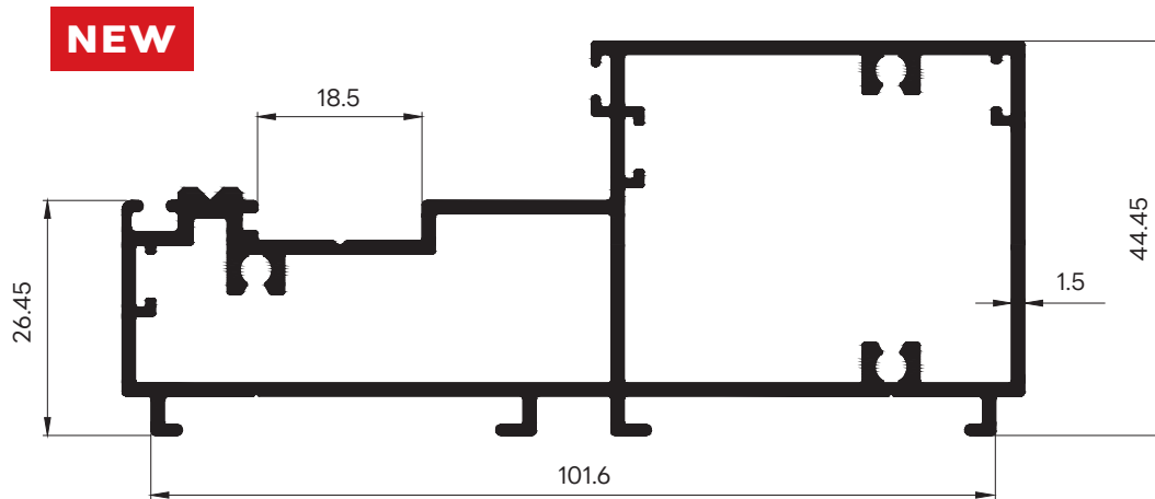
30355 WT : 1.596 Kg./m. เฟรมประตูบานเปิด
