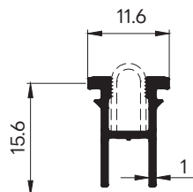
43250 WT : 0.129 Kg./m. ตัวตบหัวราง สแตนเลส
