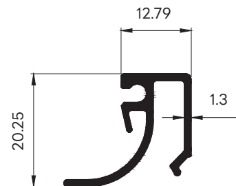
30265 ( GL 24 mm.) WT : 0.253 Kg./m. ตัวบานเปิดร่อง 29.4 มม.
