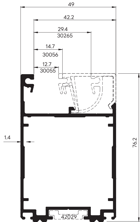
30508 WT : 1.230 Kg./m. กรอบบานพับมูเทนสไลด์
