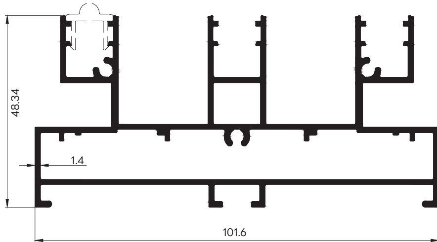
30425 WT : 1.784 Kg./m. สามรางบานเลื่อนยูโร 4 นิ้ว
