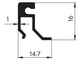
42970 (GL 8 mm.) WT : 0.159Kg./m. คิ้วกรอบบาน 3 นิ้ว
