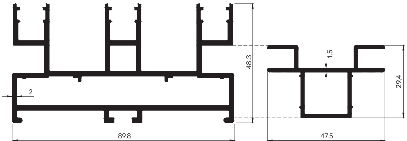
42837 WT : 2.197 Kg./m. ເຟຣມ 3 ຮາງ ລັດປັດ (89.8 ມມ.)
