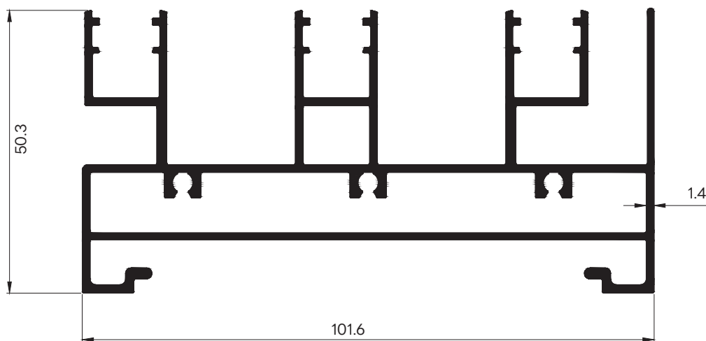
43211 WT : 1.959 Kg./m. สามรางบานเลื่อนยูโร 4 นิ้ว กันตก
