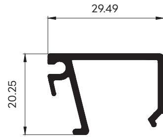
30055 ( GL 6 mm.) WT : 0.315 Kg./m. ตัวบานเปิดร่อง 12.7 มม.
