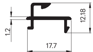
20007 WT : 0.131 Kg./m. เสริมมุมอลูมิเนียม
