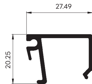
30056 ( GL 8 mm.) WT : 0.304 Kg./m. ตัวบานเปิดร่อง 14.7 มม.
