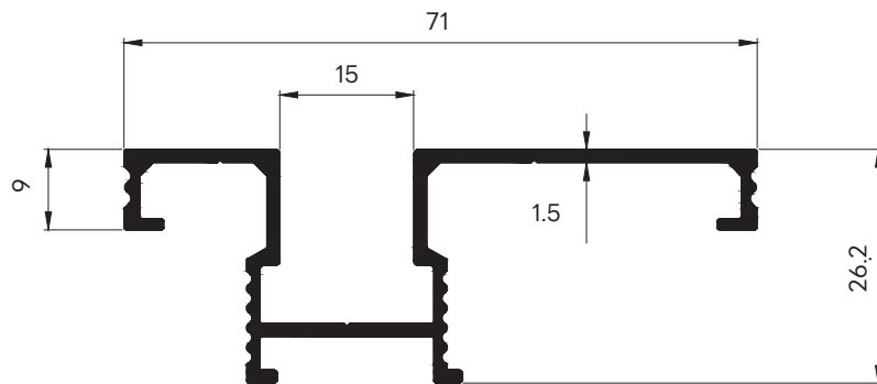
30232 WT : 0.608 Kg./m. เฟรมล่าง บานพับภายใน
