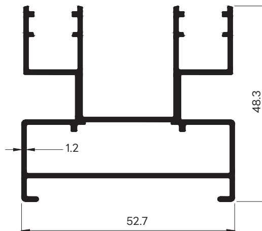
43066 WT : 0.930 Kg./m. เฟรม 2 ราง เป็ดหัว (52.7 มม.)
