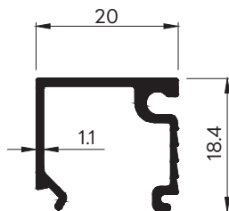
42538 (GL 6mm.) WT : 0.207 Kg./m. ຕົວຮ່ອງແສງ
