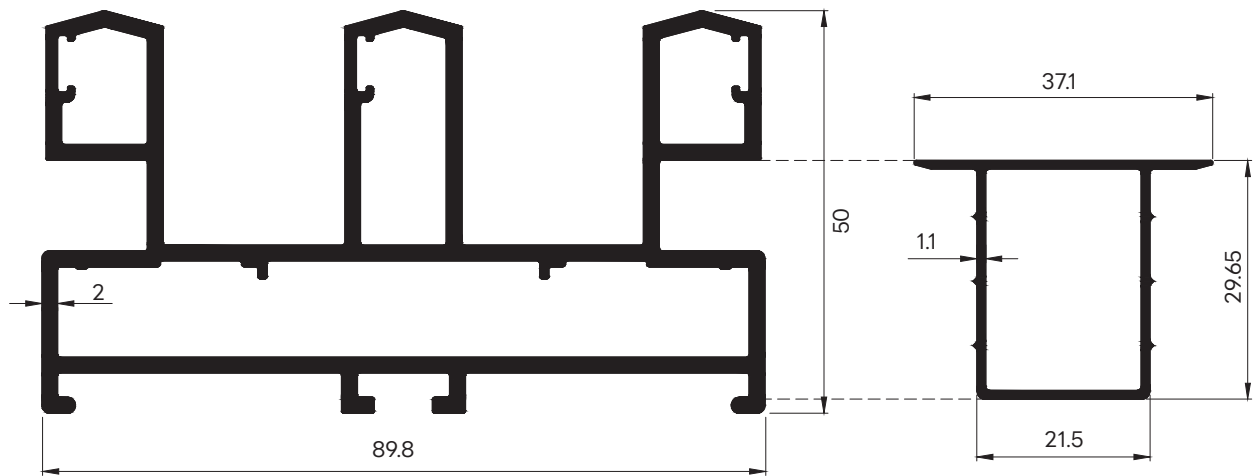
42836 WT : 2.343 Kg./m. ເຟຣມ 3 ຮາງ (89.8 ມມ.)
