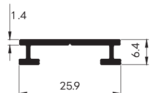
42794 WT : 0.155 Kg./m. ตัวรอง CONNECTING ROD
