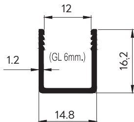
42790 WT : 0.146 Kg./m. ตัวเสริมร่องกระจก 12 มม.
