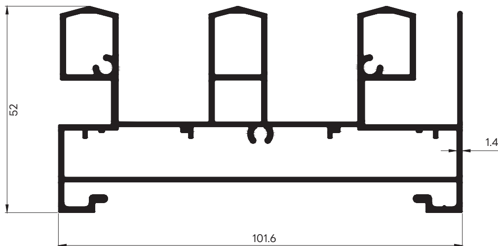
43355 WT : 2.042 Kg./m. รางยู่โรสามรางมึทึนตทหั่วปัด
