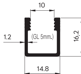
42791 WT : 0.174 Kg./m. ตัวเสริมร่องกระจก 10 มม.
