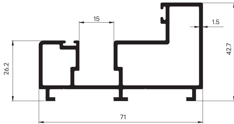
30064 WT : 1.093 Kg./m. เฟรมล่าง บานพับ
