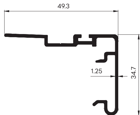
42665 WT : 0.422 Kg./m. ดุมที่ยึดบาน 3 นิ้ว
