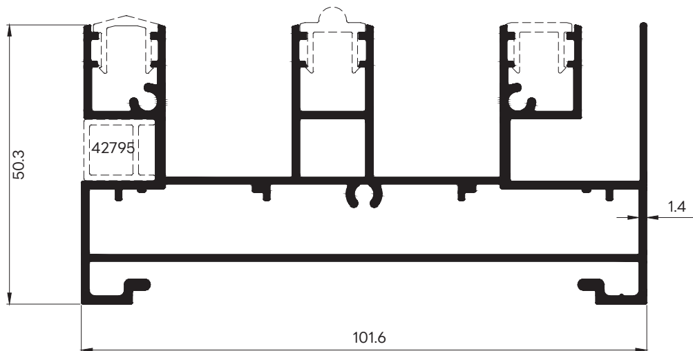
43354 WT : 1.939 Kg./m. รางยู่โรสามรางมึทึนตทหั่วปัด
