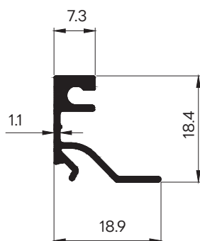
43221 (GL 20mm.) WT : 0.183 Kg./m. ຕົວກຸບຮ່ອງແສງ (25.4 ມມ.)
