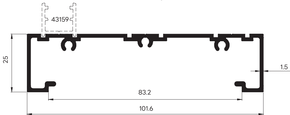
30426 WT : 0.931 Kg./m. วงกบบานเลื่อนยูโร 4 นิ้ว
