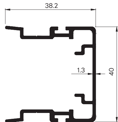
42446 WT : 0.573 Kg./m. ดุมที่ยึด 2 ทาง
